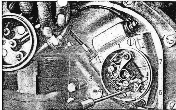
Bild 9. Unterbrecher
