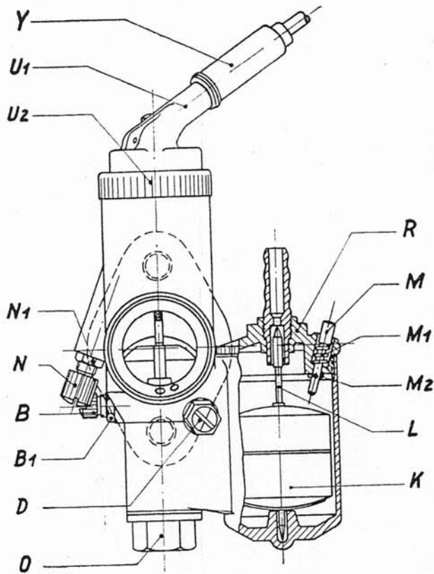
Bild 18. Vergaser R 71
