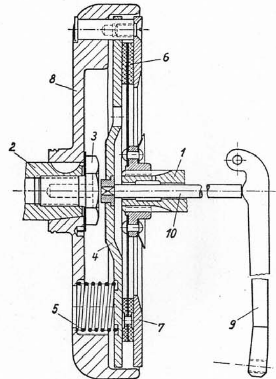
Bild 19. Kupplung
