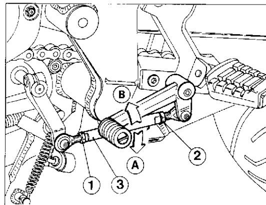
1-2) Controdado / Counternut / Contre-écrou / Gegenmutter / Contra tuercas 3) Astina / Rod / Tige / Stange / Barrila
