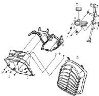
F13 ELECTRICAL,1
