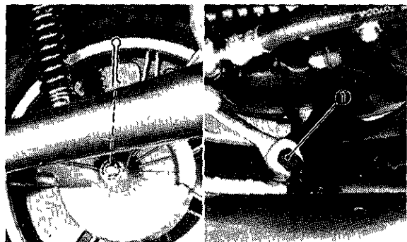
1 Pinch bolt 1 Boulons de pincement 1 Pernos de espalón
